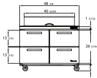
BLMT48-D4-HC
