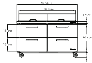
BLMT60-D4-HC
