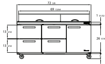
BLMT72-D4LM-HC
