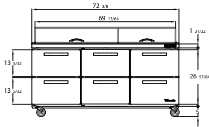
BLMT72-D6-HC
