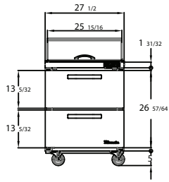
BLMT28-D2-HC
